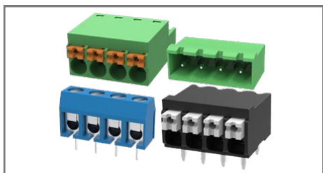
ШТЕПСЕЛЬНЫЕ, ВИНТОВЫЕ И ПРУЖИННЫЕ КЛЕММНИКИ НА КАБЕЛЬ, ПЛАТУ
